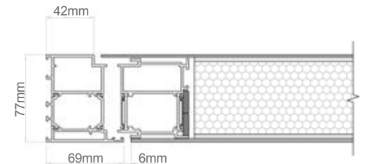
Side Jamb detail
