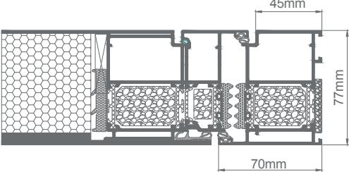
Side jamb detail
