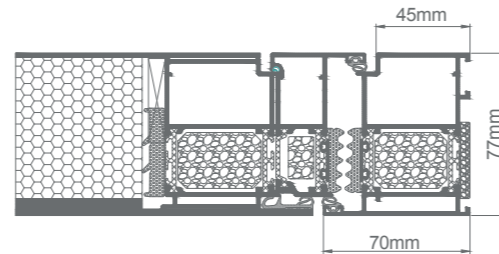
Side jamb detail
